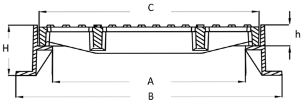
Σχέδιο τομής σχάρας
