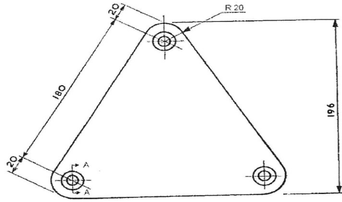
Τρίποδο ηλεκτροδίου
