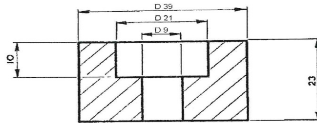
Κυλινδρικό πόδι ηλεκτροδίου Τομή Α- Α
